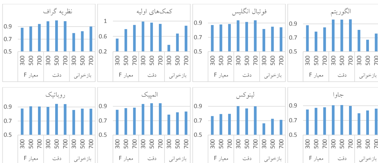
شکل ۷. میزان کارایی رده‌بندی متن بر اساس معیارهای بازخوانی، دقت و معیار F
