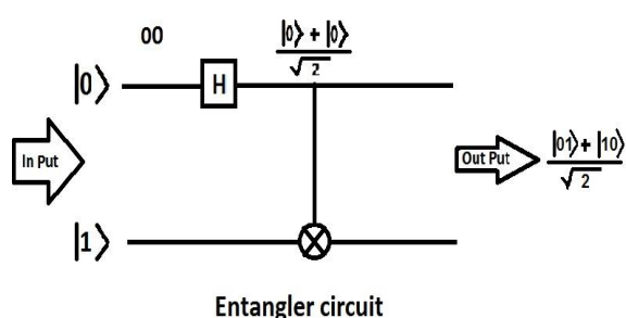
تصویر (2) مدار کوانتومی درهمتیدگی
