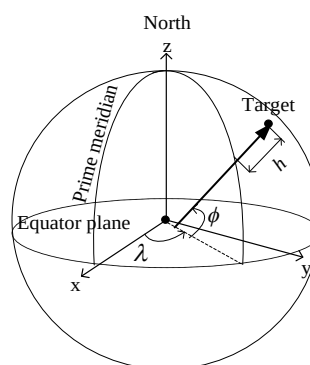
شکل 2: نمایش چارچوب مختصات ECEF کارتزین و ژئودتیک.
