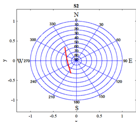
شکل 13: مشاهدات سمت -ارتفاع ماهواره از دید حسگر S_2 .
