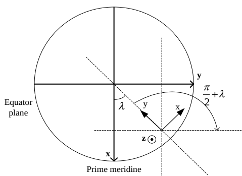
شکل 9: تصویر از بالای سیستم مختصات ECEF که در آن تصویر صفحه xy مختصات حسگر منطبق بر صفحه استوای زمین است و جهت محور y آن نیز به طرف مرکز زمین می‌باشد.
