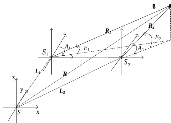
شکل 6: نمایش بردارهای هدف از دید دو حسگر غیرفعال S_1 و S_2 نسبت به مختصات مرجع S .
