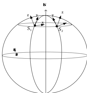
شکل 7: نمایش موازی نبودن محورهای مختصات سمت-ارتفاع دو حسگر غیرفعال به دلیل تلاقی محور y آنها در شمال زمین و وجود انحناى زمین.
