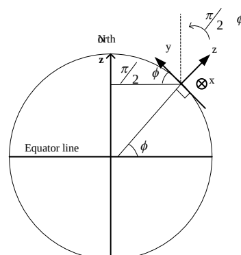
شکل 8: چرخش حول محور x مختصات سمت-ارتفاع حسگر به منظور موازی کردن محور z آن با محور z مختصات ECEF.
