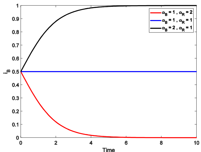
شکل (5): پاسخ مدل دینامیکی آگاهی وضعیتی دفاع سایبری فعال برای حالات مختلف قدرت مدافع و مهاجم
