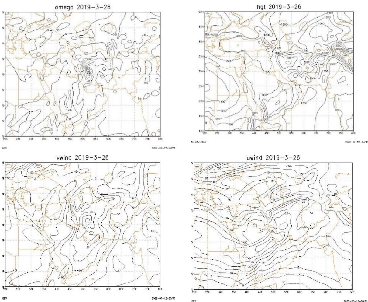
شکل 7- ارتفاع ژئوپتانسیل تراز 1000 و سرعت قائم هوا، مؤلفه مداری و نصف النهاری تراز 500 هکتوپاسکال
