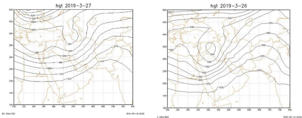
شکل 6- ارتفاع ژئوپتانسیل تراز 500 هکتوپاسکال
