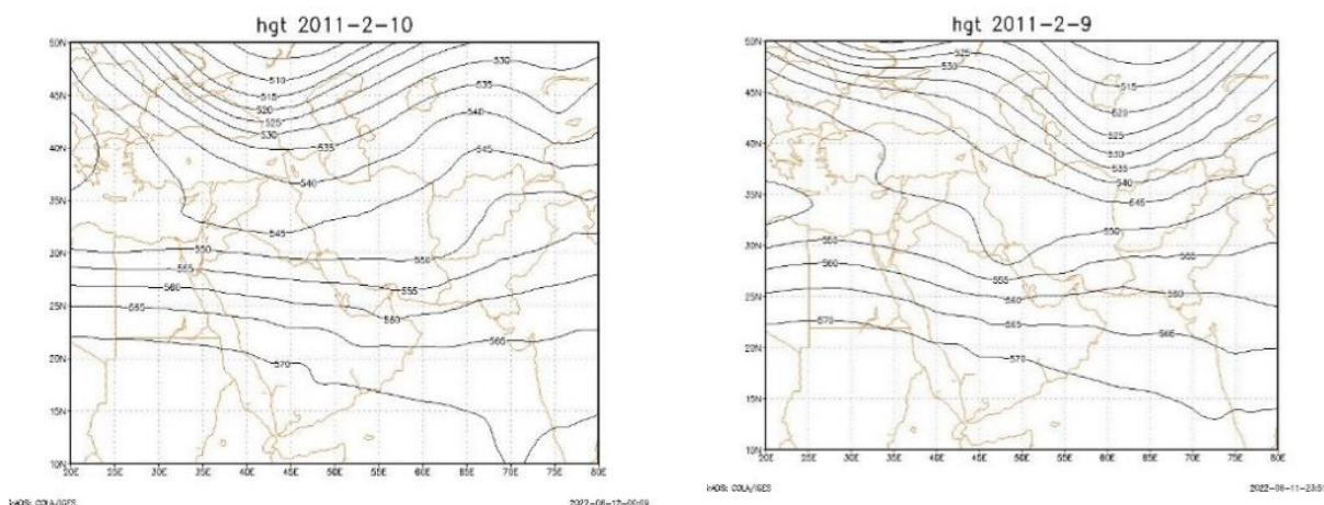
شکل 4- ارتفاع ژئوپتانسیل تراز 500 هکتوپاسکال
