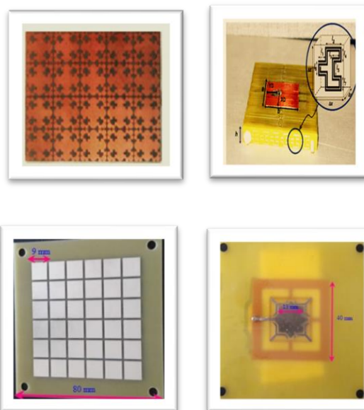
شکل (۶). ساخت برد و آنتن بچ روزنه ای.
