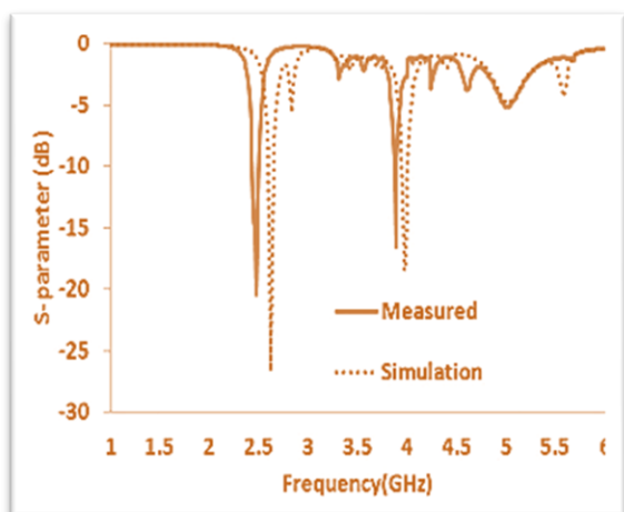
شکل (۷). پارامتر پراکندگی شبیه سازی و اندازه گیری شده آنتن پیشنهادی بچ روزنه ای.
