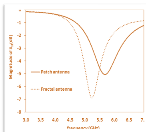
شکل (۹). تلفات بازگشتی برای پچ و آنتن فراکتال
