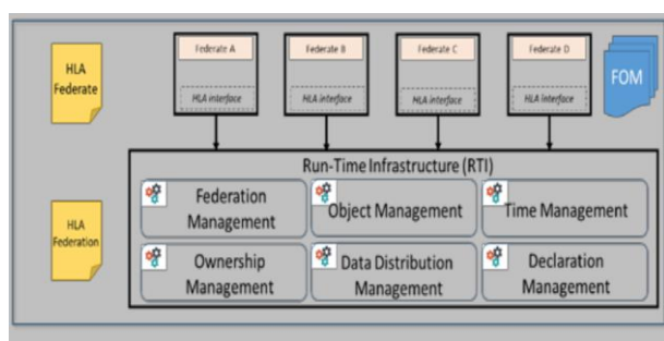
شکل ۴: نمودار HLA
